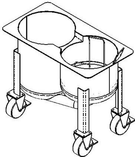
fahrbares Tauchbecken
