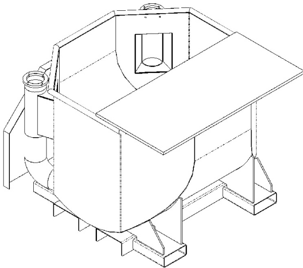
Rührwerksbehälter 1000 Liter
