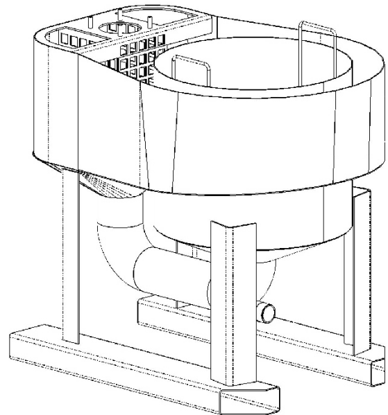
Tauchbecken
