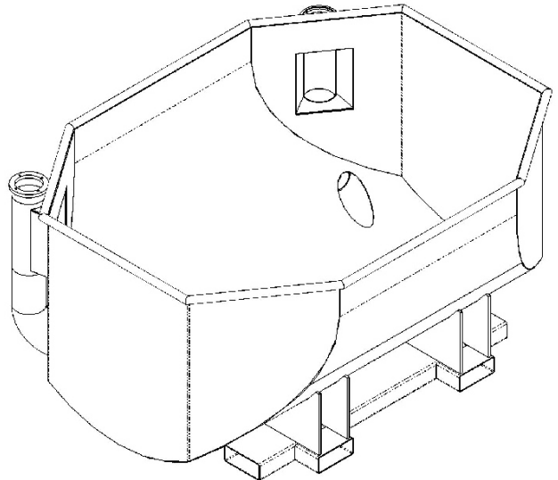
Tauchbecken mit Auffangwanne
