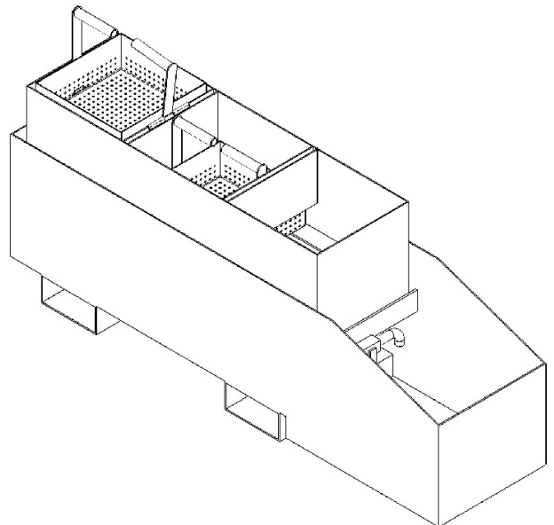
Tauchbecken mit Auffangwanne
