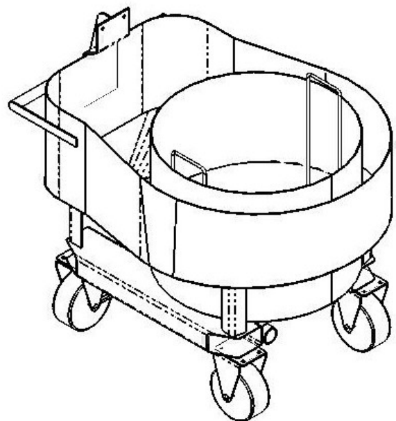
fahrbares Tauchbecken Ø700mm
